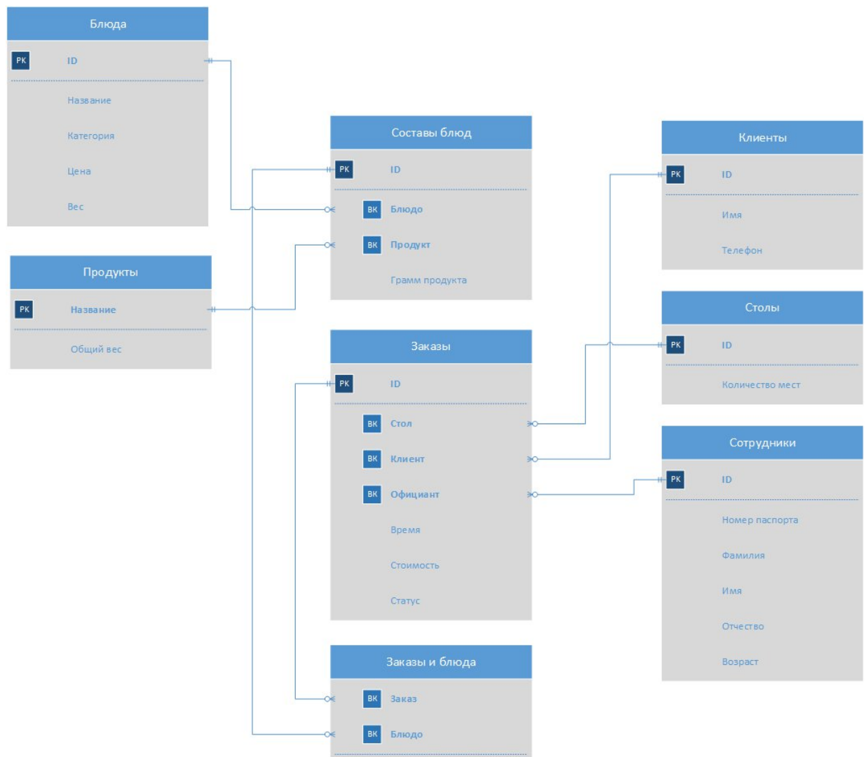
Рисунок 1 – ER-модель
